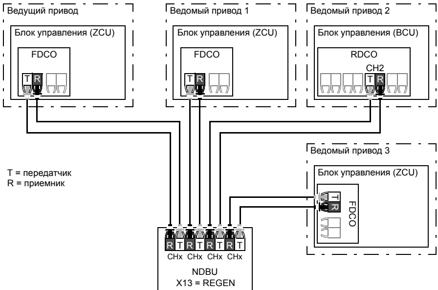
Схема "звезда" (2)
