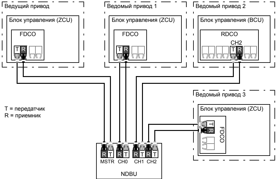
Схема "звезда" (1)
